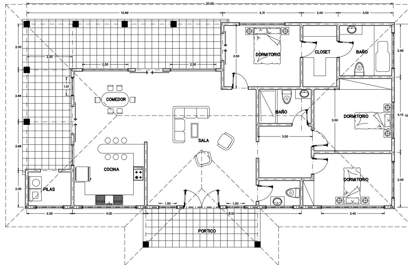
PLANTA DE DISTRIBUCION ARQUITECTONICA ESC.1:50
