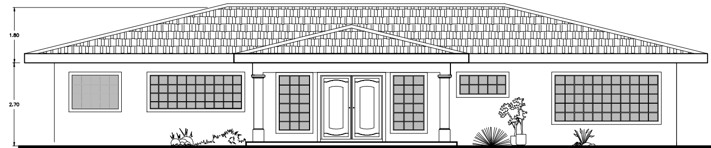
ELEVACION PRINCIPAL ESC.1:50
